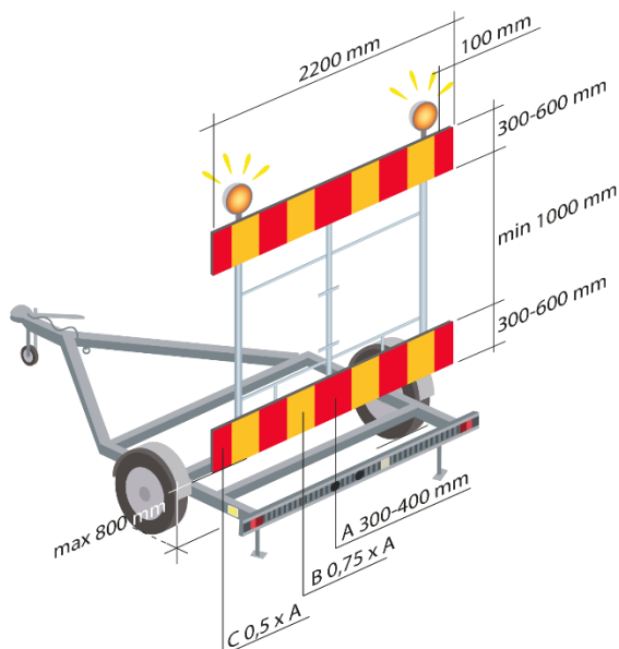
Illustration 9.5.1.1 Vägmarkesvagn
