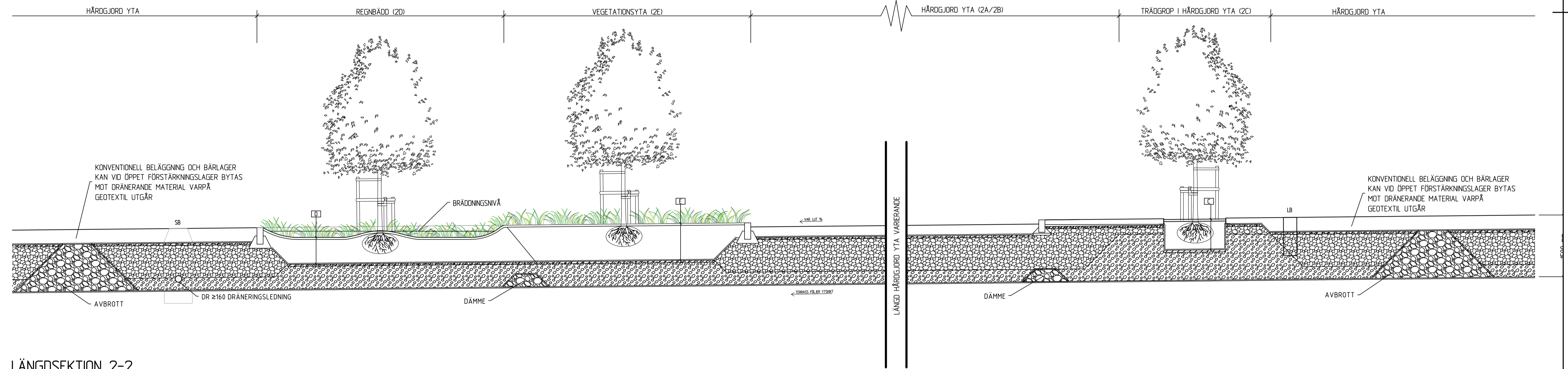
LÄNGDSEKTION 2-2 SAMMANHÄNGANDE STRÅK 2A, 2B, 2C, 2D & 2E SKALA A1 1:50, A3 1:100
