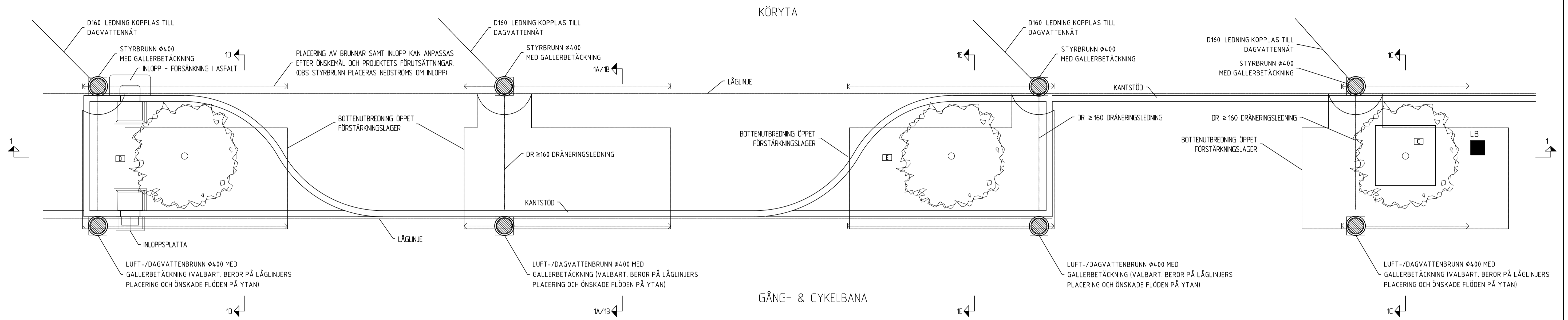
PLAN ENSKILDA KONSTRUKTIONER 1A, 1B, 1C, 1D & 1E SKALA A1 1:50, A3 1:100
