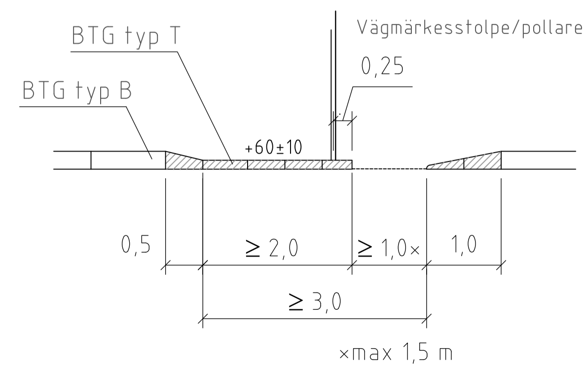
BETONGKANTSTÖD Skala: 1:50
