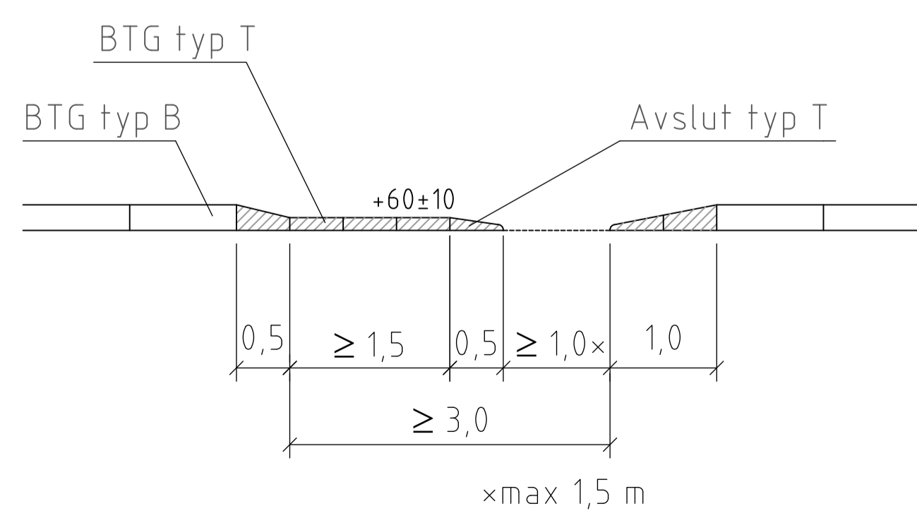
BETONGKANTSTÖD Skala: 1:50
