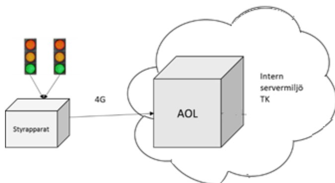
Figur 2 – Systemarkitektur Kommunikation
