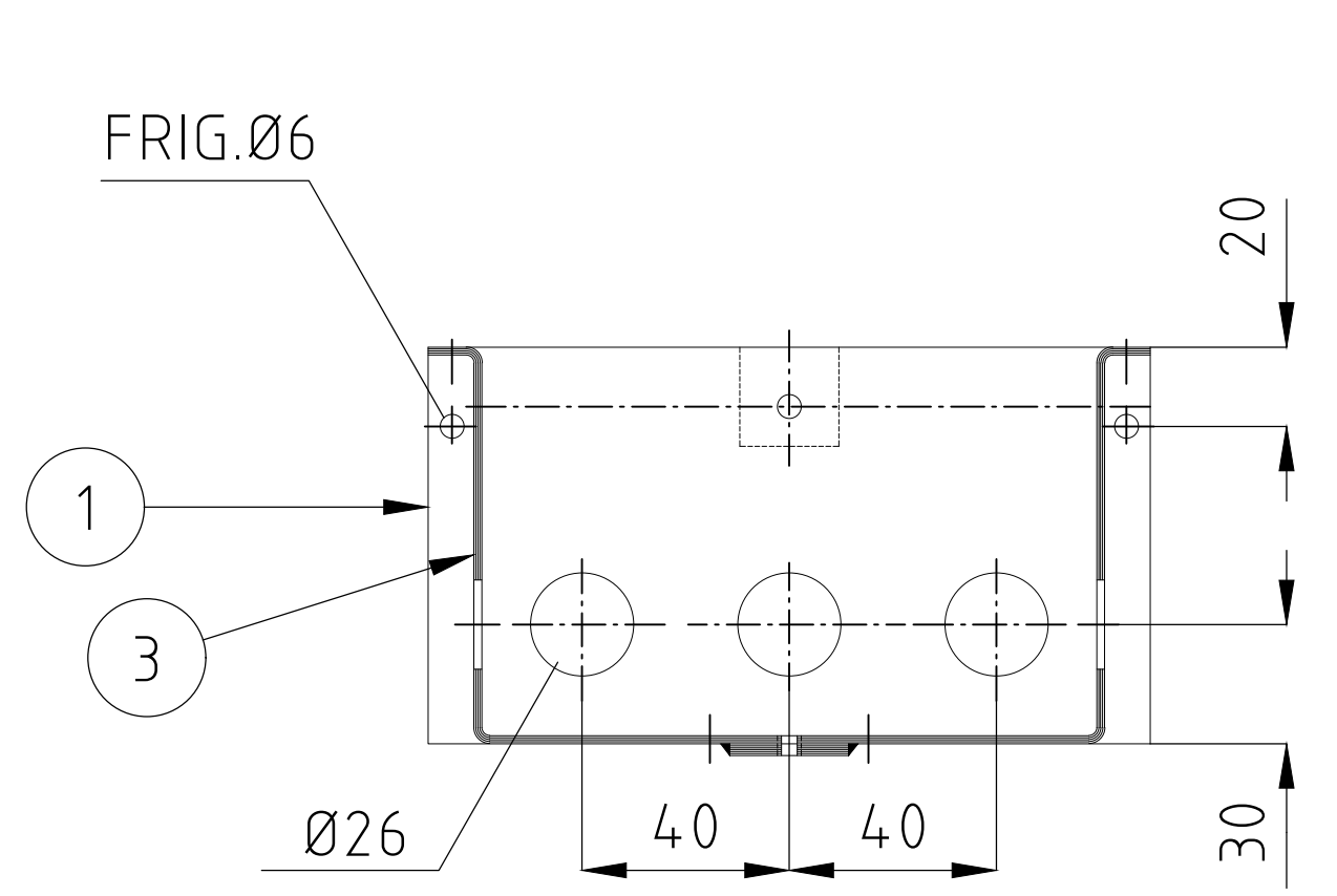
A - A1 Topp
