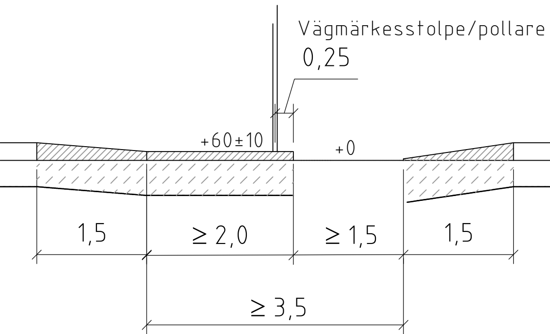
SEKTION B - B GRANITKANTSTEN Skala: 1:50
