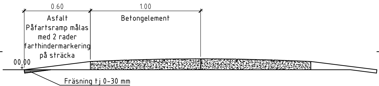
SEKTION A-A SKALA 1:20
