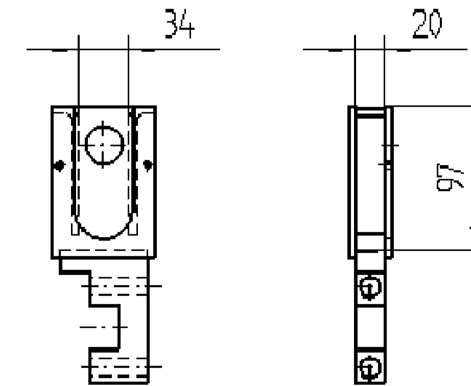
Abmessungen Stelleisentasche M 1:5
