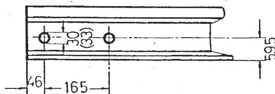
Detaljhålning för skarvjärn Skala 1:10 Schienenlochung 33 mm \phi ab 30-m-Schienen
