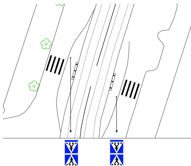
Bild 24. Principskiss över Plantagegatans spårövergång
