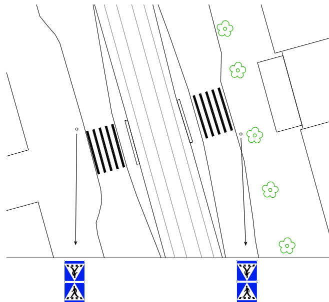
Bild 36. Principskiss över Postgatans spårövergång
