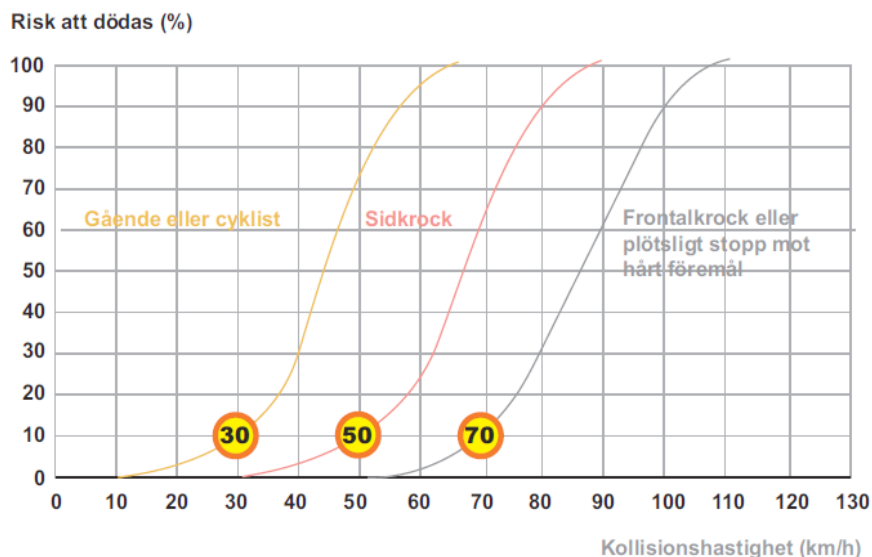
Bild 1. Krockvåldskurvor
