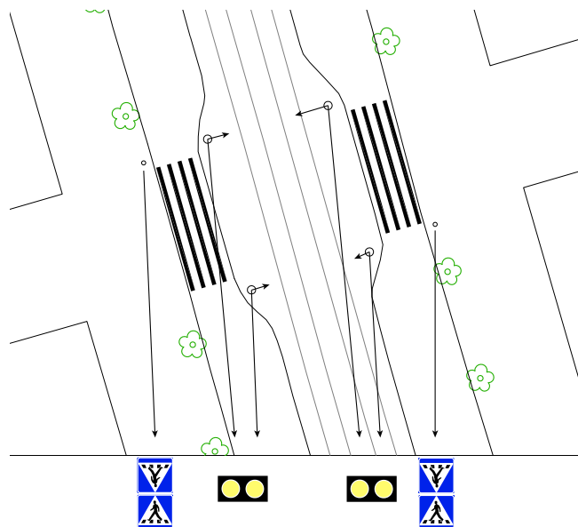
Bild 30. Principskiss över Kungsgatans spårövergång
